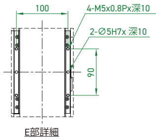
E部詳細
