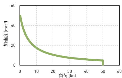
加速度-負荷曲線
