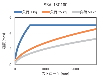
速度-ストローク曲線
