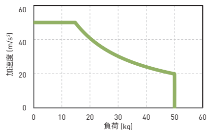
加速度-負荷曲線
