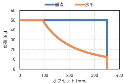
偏心負荷容量曲線
