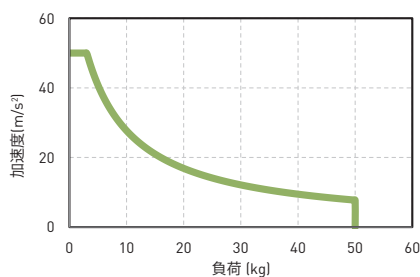
加速度-負荷曲線
