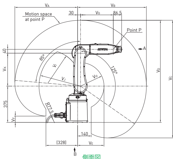
側面図
