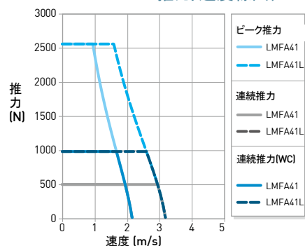
■ 推力/速度線図( DCバス電圧 = 325 V DC )
