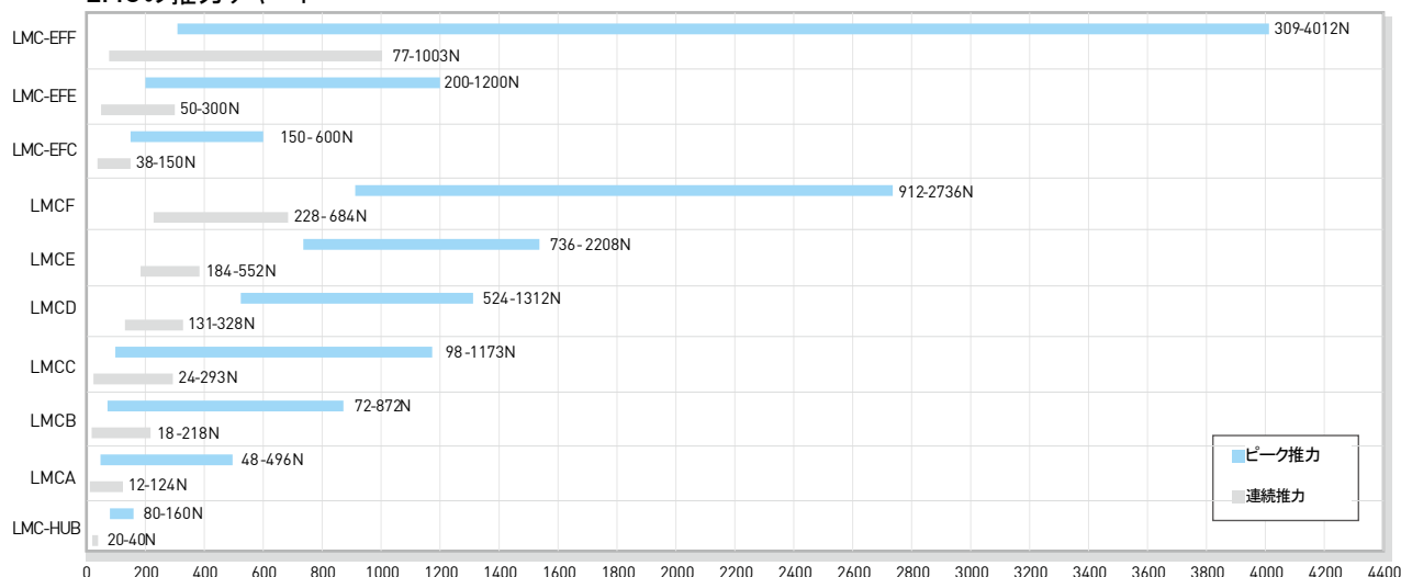
LMCの推力チャート
