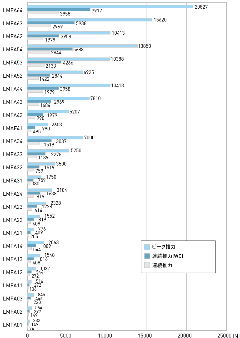
LMFAの推力チャート
