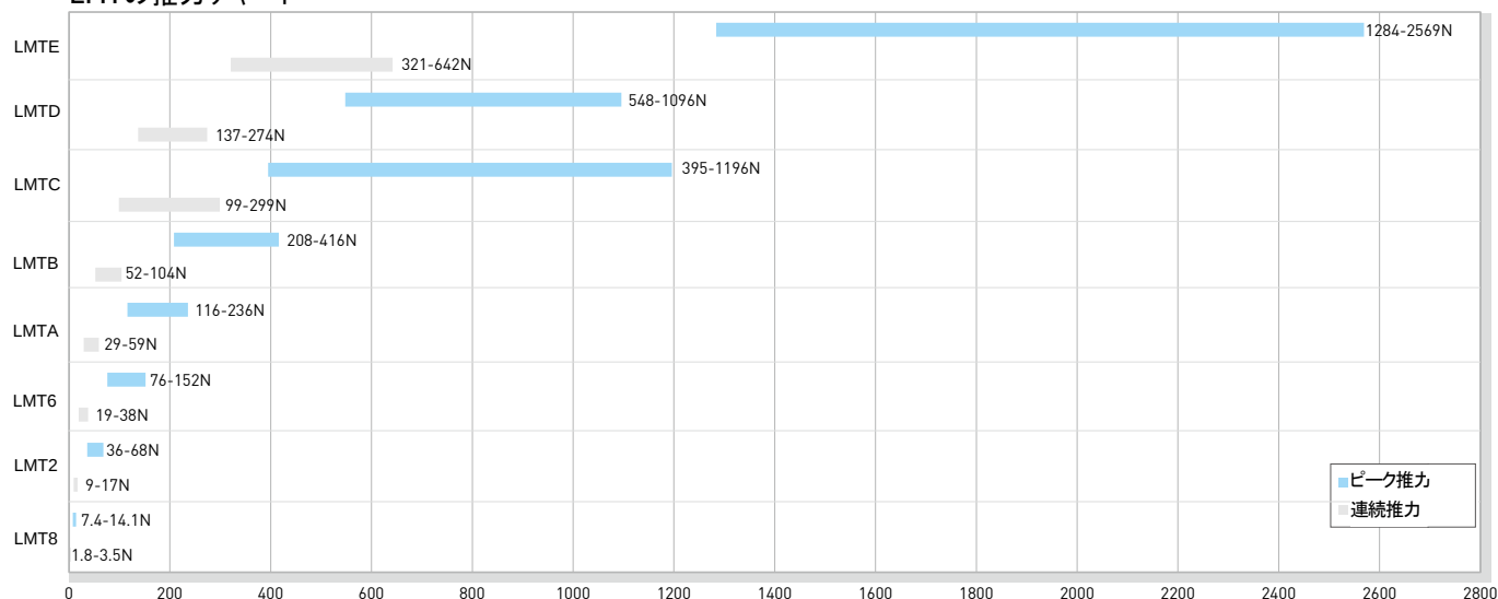
LMTの推力チャート
