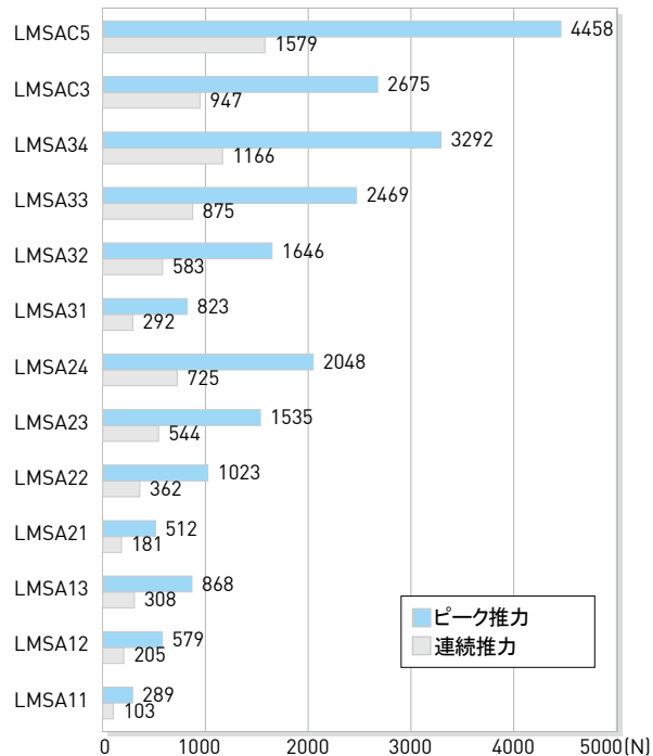
LMSAの推力チャート
