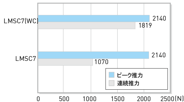
LMSCの推力チャート
