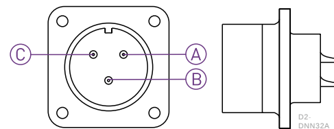
WPS3102A14S-7P-R
