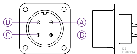
WPS3102A18-10P-R
