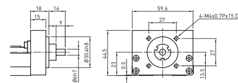
アダプタブラケット H1
