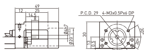
モータフランジ F1
