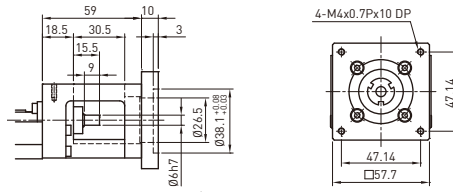
モータフランジ F5
