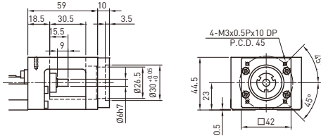
アダプタブラケット H0
