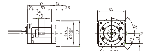
モータフランジ F5
