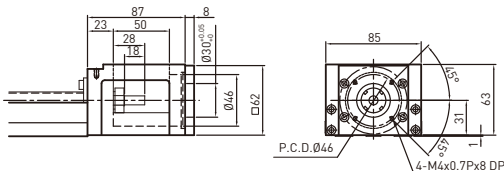
モータフランジ F3
