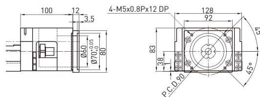
アダプタブラケット H0
