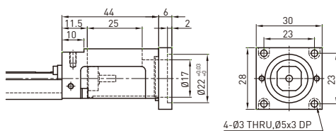
モータフランジ F3
