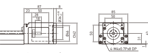
モータフランジ F6
