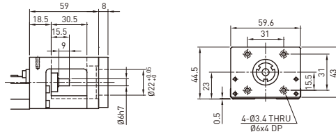
アダプタブラケット H1
