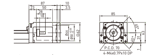
モータフランジ F2
