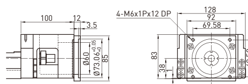
モータフランジ F4
