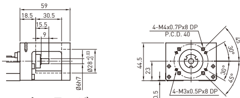
モータフランジ F1
