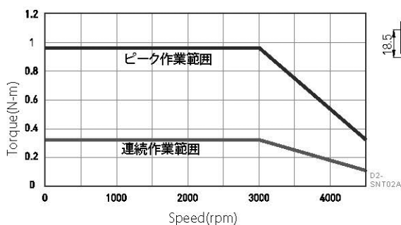
FRLS 100W トルク-回転速度曲線
