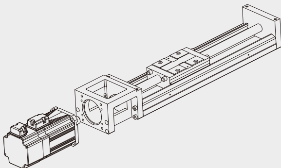
ロボット - サーボモータ接続
