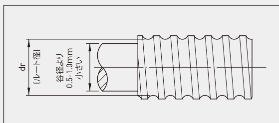
図4.7：内部循環式ボールねじのエンドジャーナルの特殊仕様
