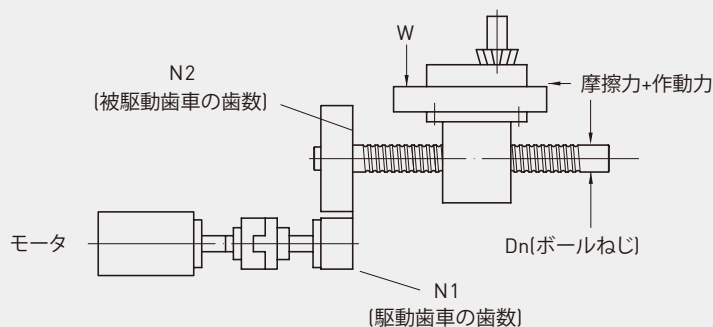
図4.23：ボールねじによる荷重動作
