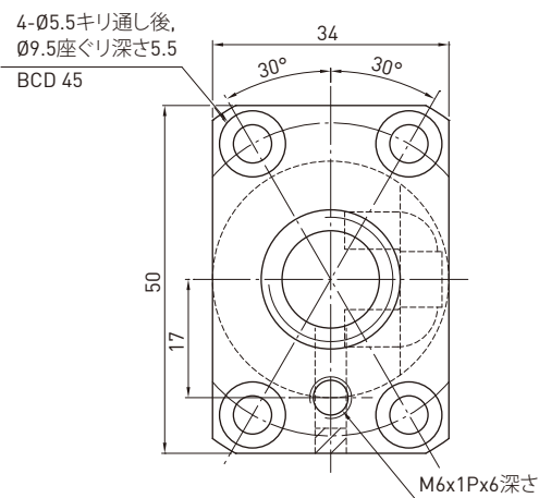
D-D 矢視
