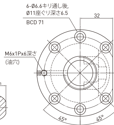
D-D 矢視
