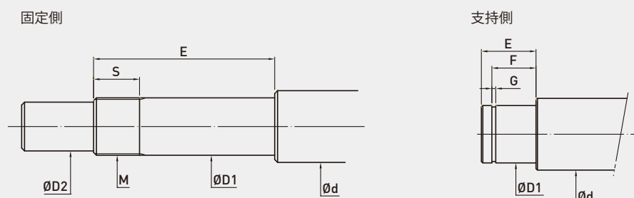
図3.5：ねじ軸軸端の形状
