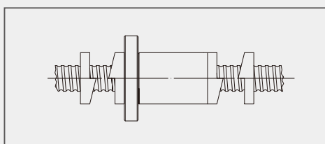
図4.5：ナットのオーバトラベルを防止する為のドッグストップ
