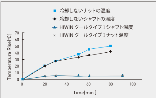
図8.4：クールタイプIボールねじ昇温のテスト (Dm-N=150,000)
