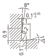
X 詳細図
