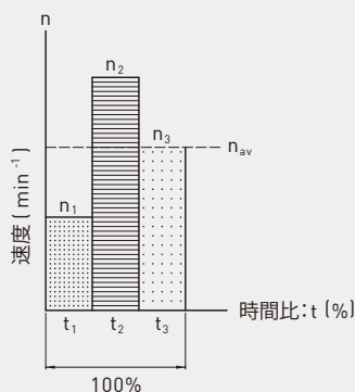
図4.22：等価速度
