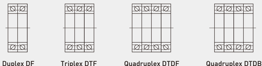
図4.4：ボールねじサポートベアリングの各種の組合わせ
