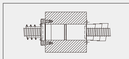
図4.6：テレスコピック又はベローズタイプカバーによるボールねじの防護
