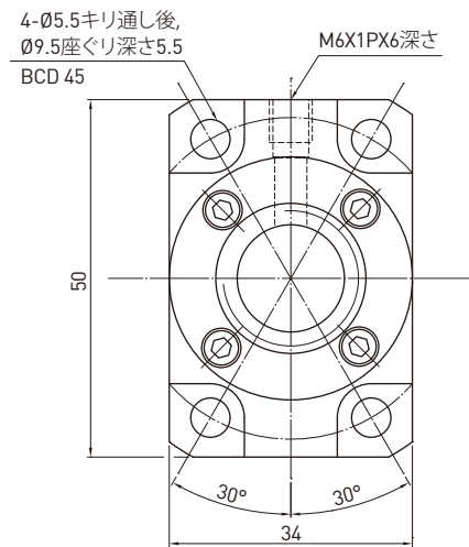
D-D 矢視
