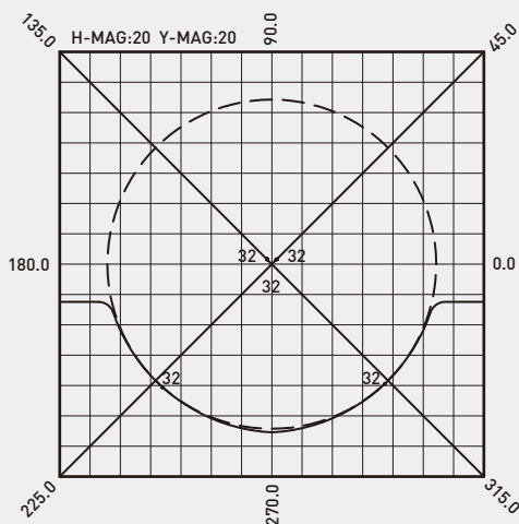
図2.4：プロファイルレーサによるねじ溝形状のチェック
