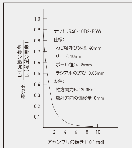
図4.3(b): ラジアル荷重による疲れ寿命の影響
