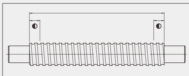
図4.8：ボールねじ部の熱処理の領域
