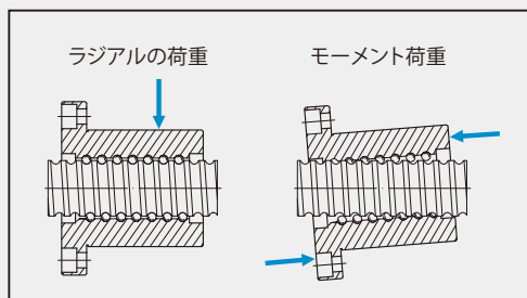
図4.3(a): 取付誤差の影響
