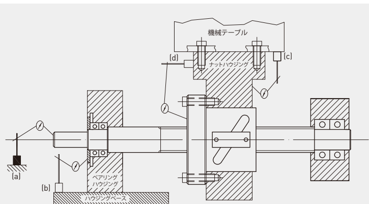
図A.4：異常バックラッシュの原因の追跡
