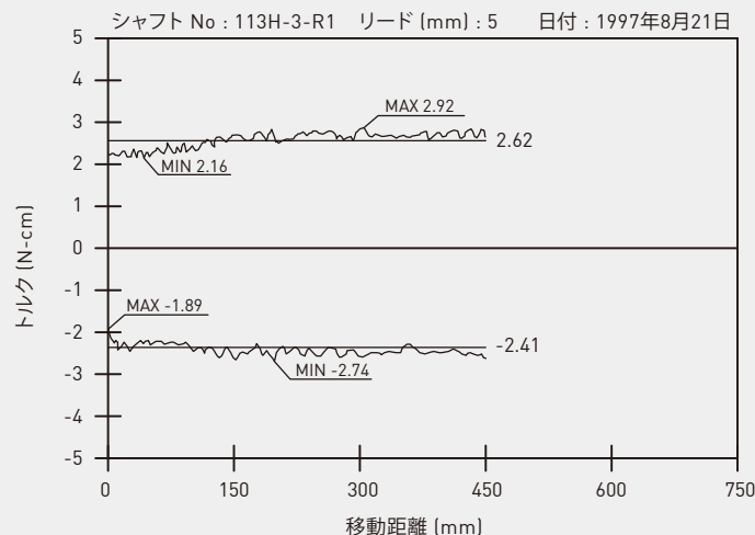
図2.5：HIWIN 予圧チェックダイアグラム
