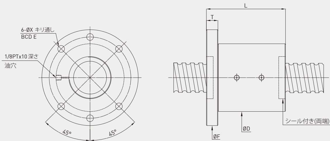
カセット式重負荷ボールねじ寸法表 (FSC)
