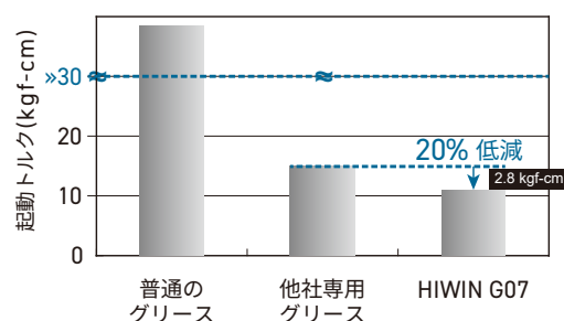
-40°C時で異なるグリースの起動トルク比較
