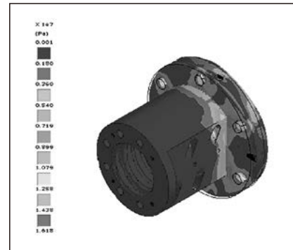
図8.10：FEM分析によるボールねじ
