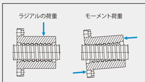
図4.3(a): 取付誤差の影響 ボールねじの支持部(ねじ軸、支持軸受、案内など)の取付が一直線になっていない時、偏心荷重が加わると、作動性に悪影響を及ぼします。
