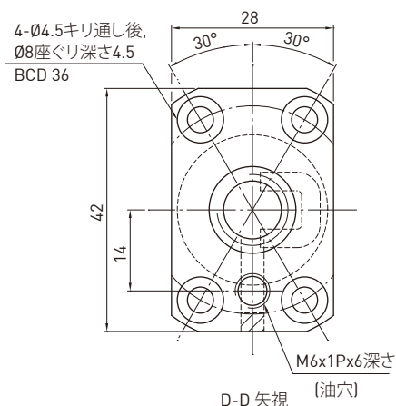
D-D 矢視
