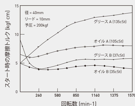
図4.32：油の粘度高と摩擦トルクとの関係
