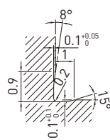
F0.2X0.1DIN509 X 詳細図
