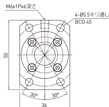
D-D 矢視
