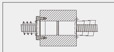
図4.6: テレスコピック又はベローズタイプカバーによるボールねじの防護
