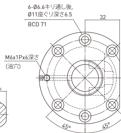
D-D 矢視
