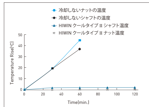
図8.9：高速運転の状況でクールタイプ II ボールねじ昇温の比較
