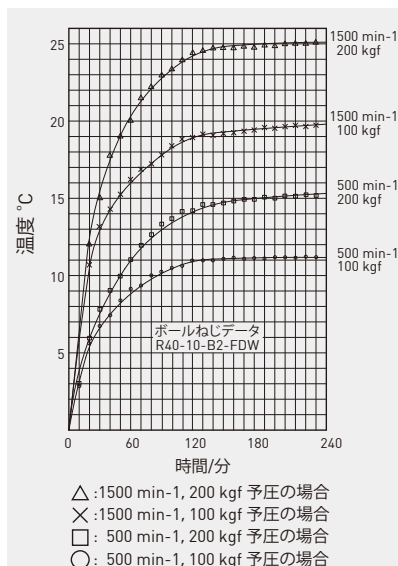
図4.30：運転速度、予圧ナットおよび昇温の関係
