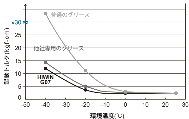
-40°C時で異なるグリースの起動トルク比較
