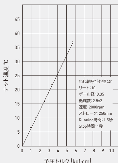
図4.31：ナットの昇温と予圧摩擦トルクとの関係
