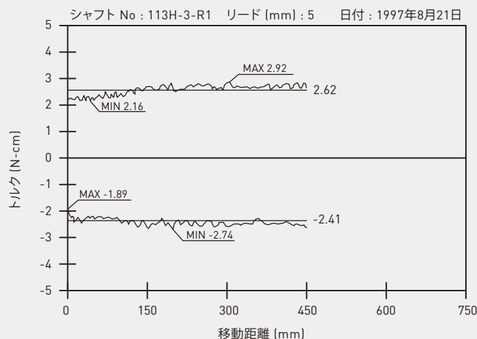
図2.5：HIWIN 予圧チェックダイアグラム
