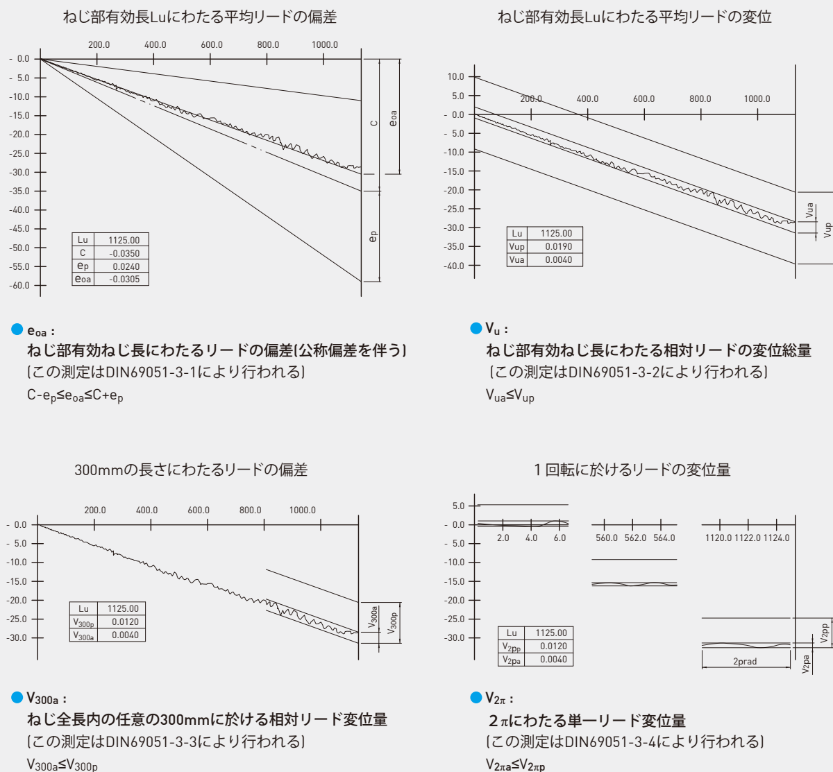
図4.14：DIN69051によるダイナミックレーザ測定機器を使用した場合のリード精度測定表
