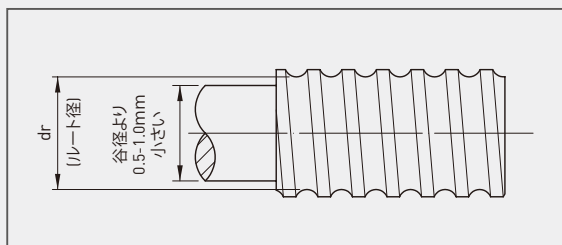
図4.7: 内部循環式ボールねじのエンドジャーナルの特殊仕様
