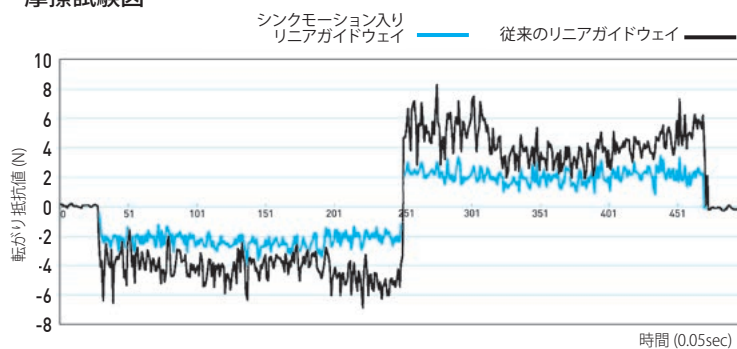
摩擦試験図
