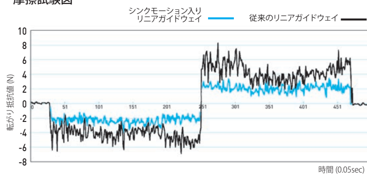
摩擦試験図
