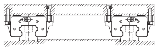
取付ボルトの方向が異なるHGW型のブロック
