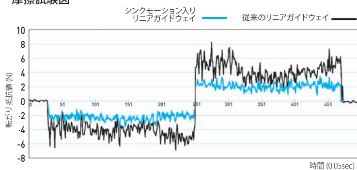
摩擦試験図
