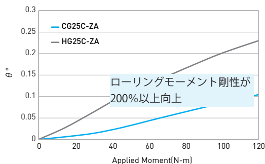
剛性テスト
