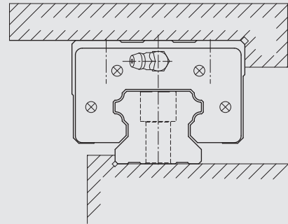
レール 1 本使用と取付基準側
